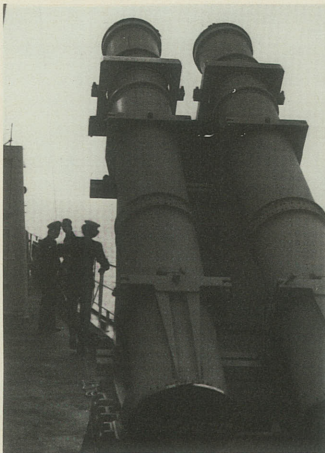
Afskydningsramper for Harpoon missiler i NIELS JUEL. Foto: Kaj Lund.
